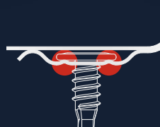
Išėmos varžtams
