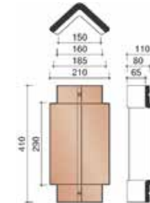
Kraigo pradžios čerpė
