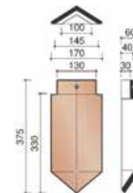
Valminio kraigo pradžios čerpė
