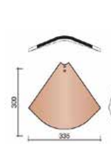
Valminio kraigo čerpė
