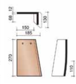
Vėjalentinė čerpė dešinė
