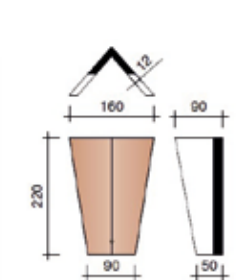
Valminio kraigo čerpė
