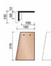
Vėjalentinė čerpė kairė
