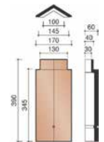
Valminio kraigo čerpė
