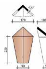
Valminio kraigo pradžios čerpė
