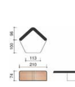
Kraigo pradžios/pabaigos dangtelis
