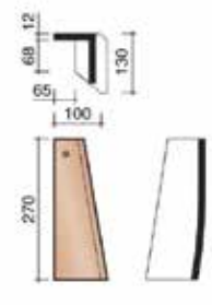
½ (pusinė) vėjalentinė čerpė dešinė
