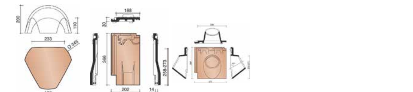
Valminė universali kraigo čerpė (Y-formos)
