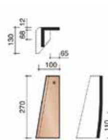
½ (pusinė) vėjalentinė čerpė kairė
