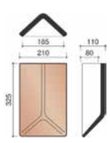
Valminė universali kraigo čerpė (Y-formos)
