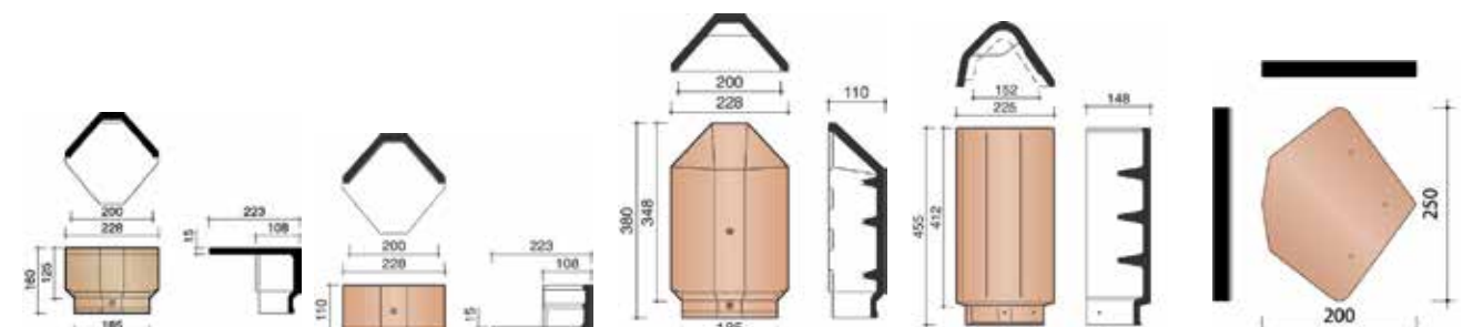
Kraigo pradžios dangtelis
