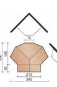
Valminė universali kraigo čerpė (Y-formos)
